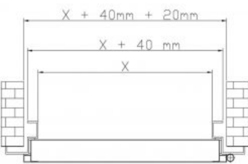
Podstawowe zależności wymiarowe Drzwi FUTRYNA KĄTOWA
