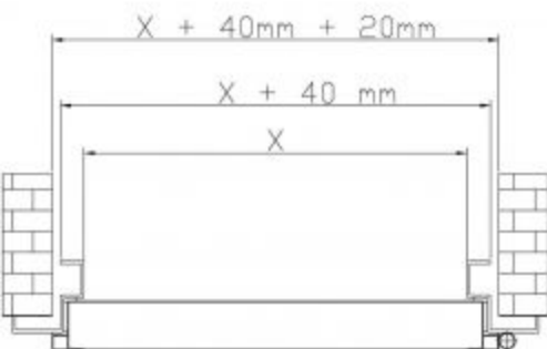
Podstawowe zależności wymiarowe Drzwi FUTRYNA KĄTOWA
