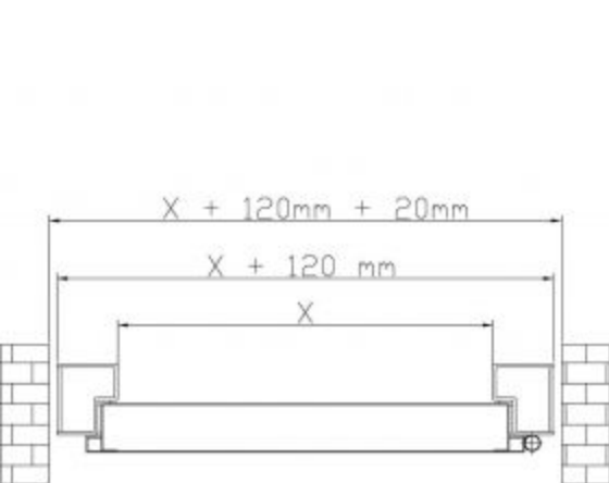
Podstawowe zależności wymiarowe Drzwi FUTRYNA CEDIWA
