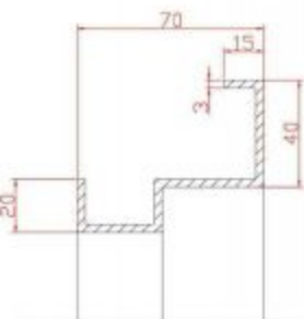
Przekrój pionowy Futryna kątowna
