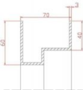
Przekrój pionowy Futryna ceowa
