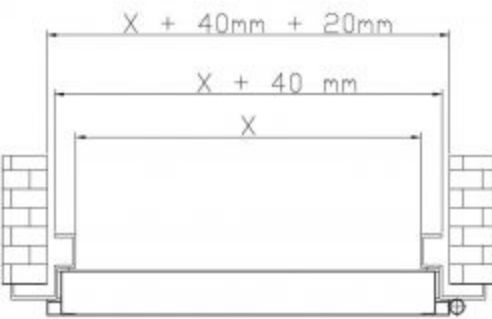
Podstawowe zależności wymiarowe Drzwi FUTRYNA KĄTOWA
