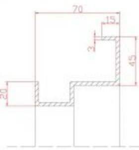
Przekrój pionowy Futryna kątowna
