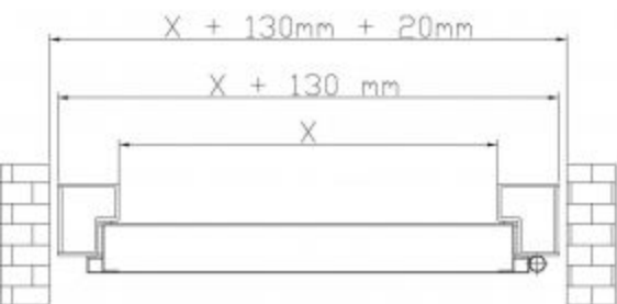
Podstawowe zależności wymiarowe Drzwi FUTRYNA CEDIWA
