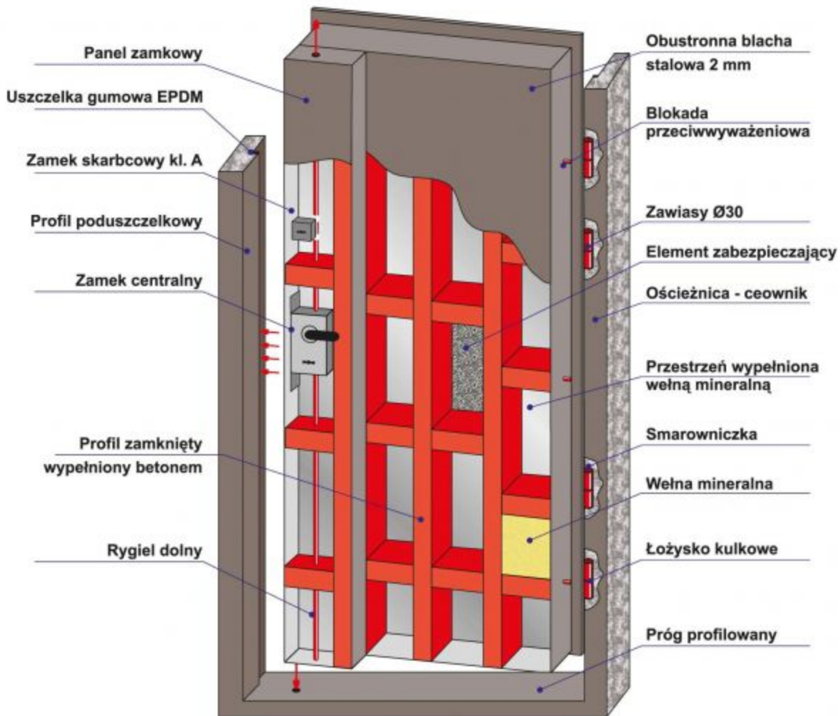
Wersja z dwustronnym dostępem klucza z wypełnieniem betonem:
