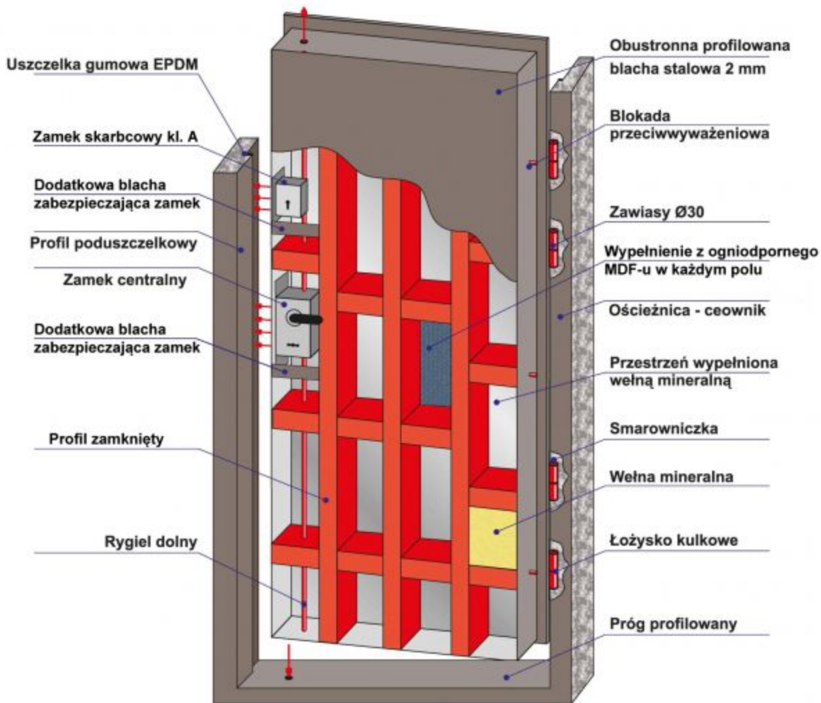
Wersja z dwustronnym dostępem klucza z wypełnieniem z ogniodpornego MDF-u:
