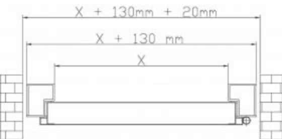
Podstawowe zależności wymiarowe Drzwi FUTRYNA CEDWA
