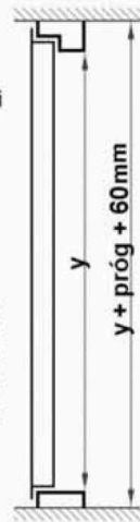
Podstawowe zależności wymiarowe Drzwi DC 3.1KT-M futryna ceowa
